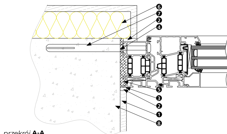
przekrój A-A
