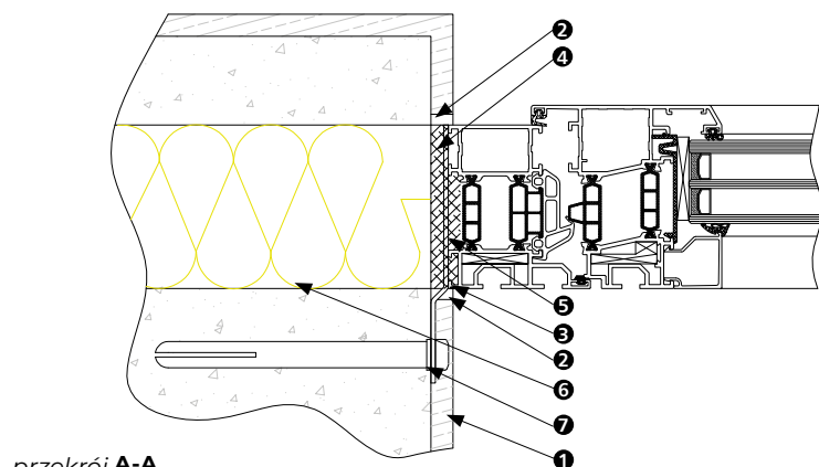
przekrój A-A
