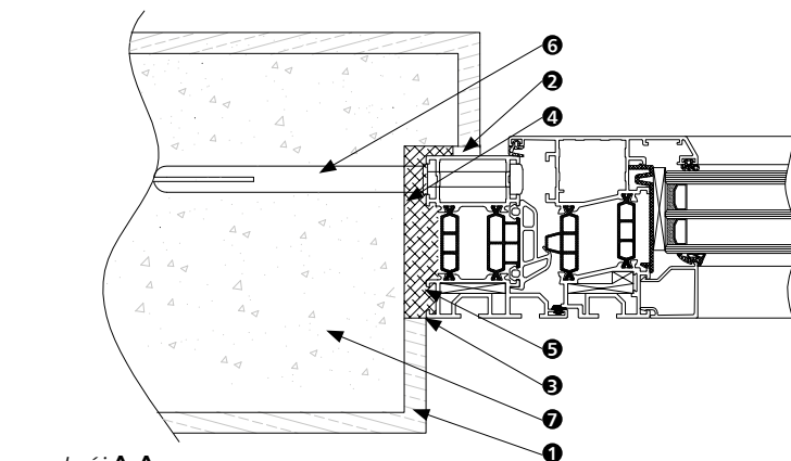
przekrój A-A
